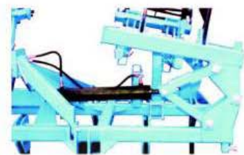
hydraulische Klappung
