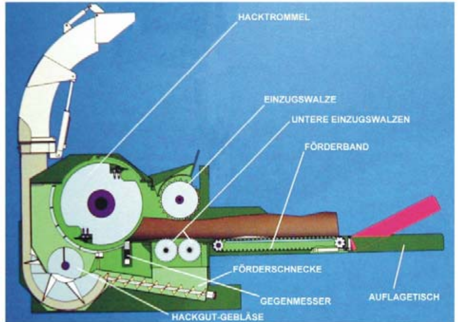
Aufbauschema
